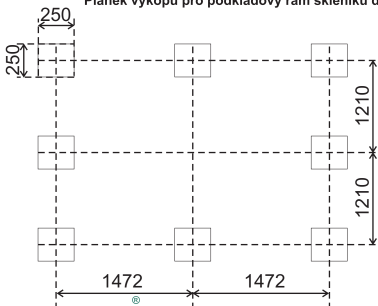
Plánek výkopů pro podkladový rám skleníků délky 3 m
