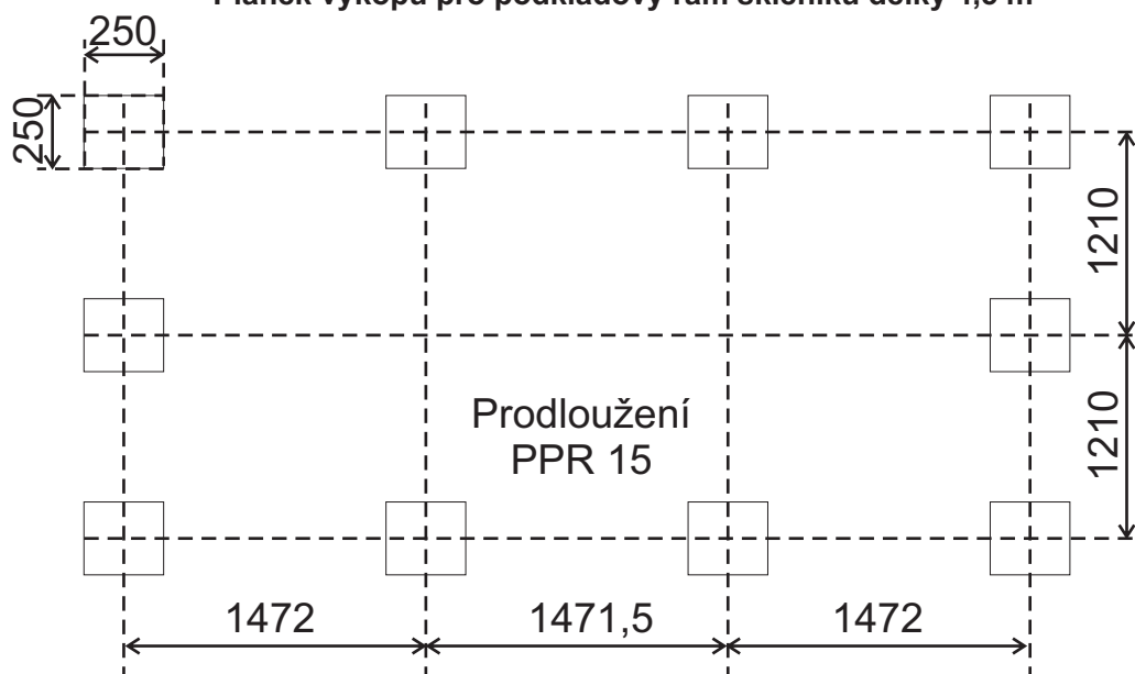
Plánek výkopů pro podkladový rám skleníků délky 4,5 m
